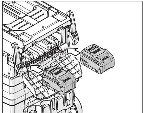
Fig. 50: Batterium med to 18-V-batterier
